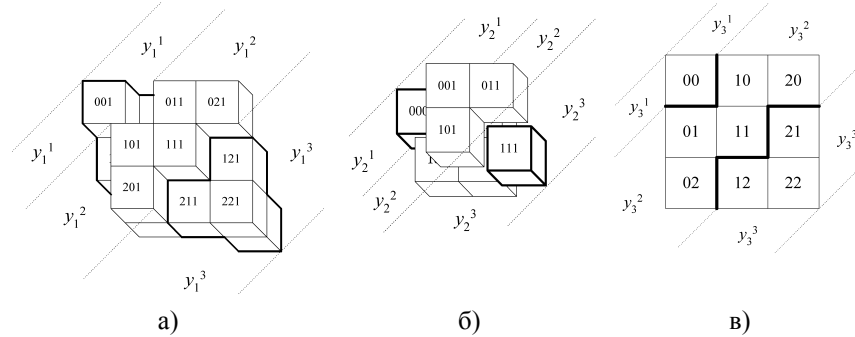
Рис. 2. Схема формирования шкал оценок для составных критериев AK_1, AK_2 и AK_3
